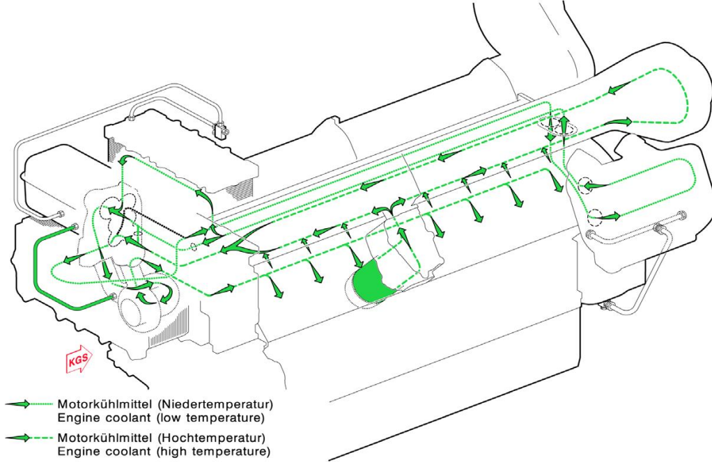
Şekil 3-39: Kapalı Tıp Soğutma
