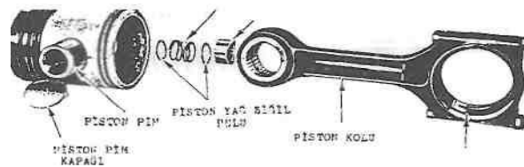
Şekil 3-22. Piston Kolu
