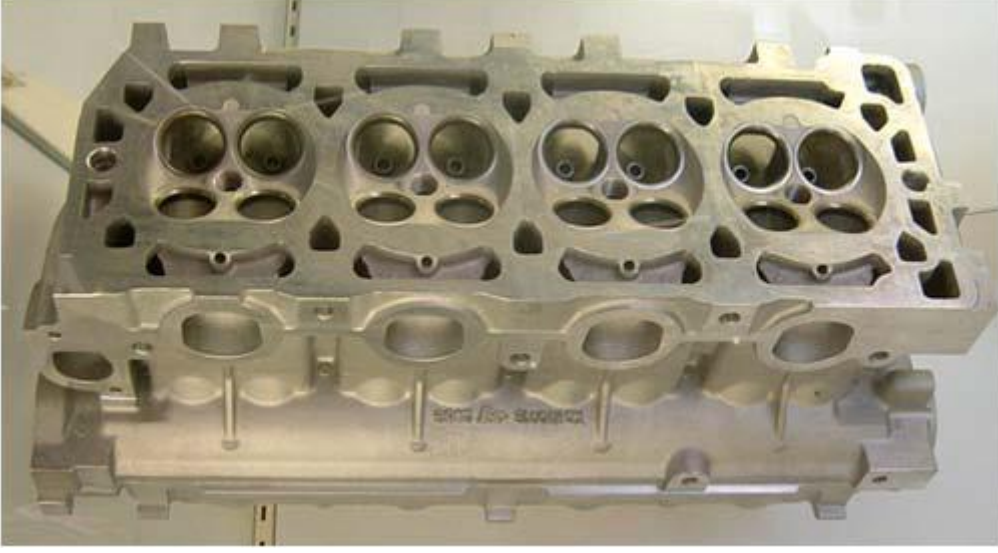
Őekil 3-7: Dört zamanlı dört silindirli bir motora ait silindir kapağının üstten görünüşü
