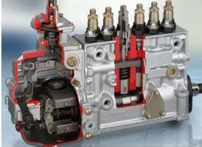
Şekil 3-51: Sıra tip pompa kesiti
