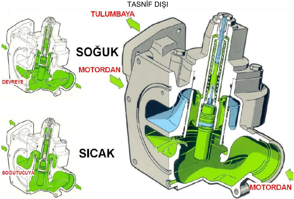
Şekil 3-42: Termostat
