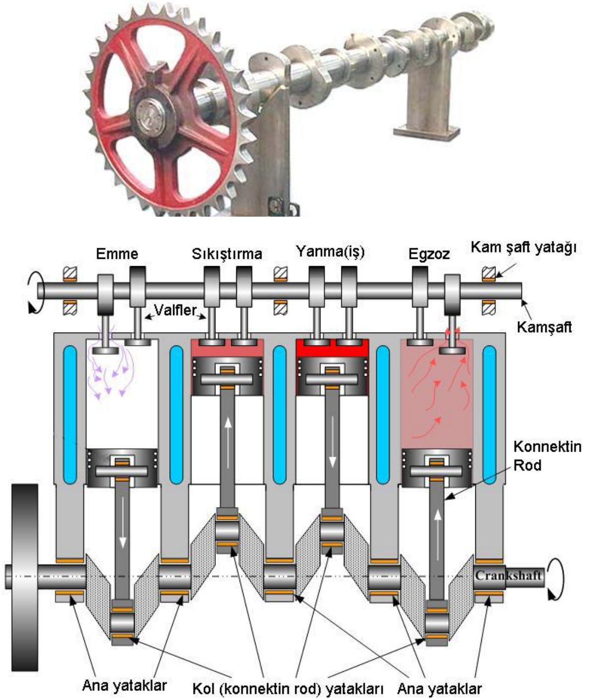
Şekil 3-25: Üstten kamlı bir motorda valf (supap) hareket mekanizması bileşenleri
