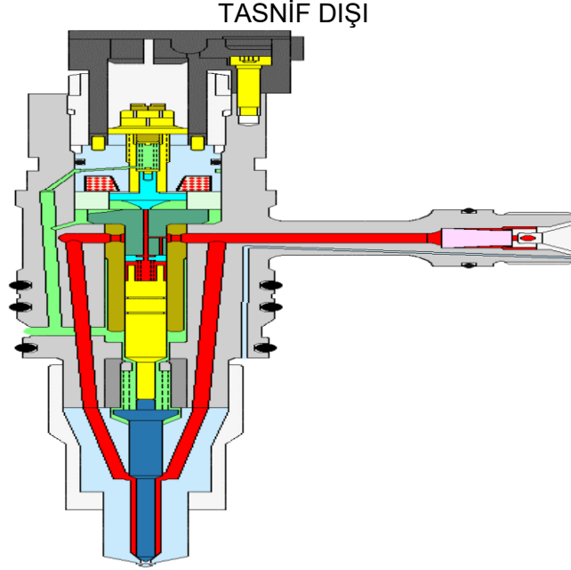
Şekil 3-52: Bosch Enjektör
