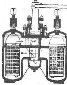
Şekil 3-48: Yakıt Streyneri
