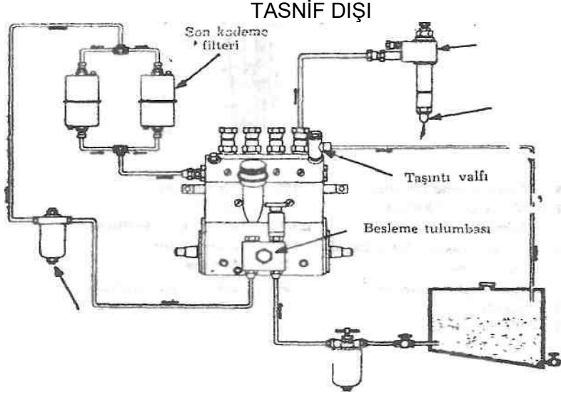
Şekil 3-50 : Bosch Yakıt Sistemi
